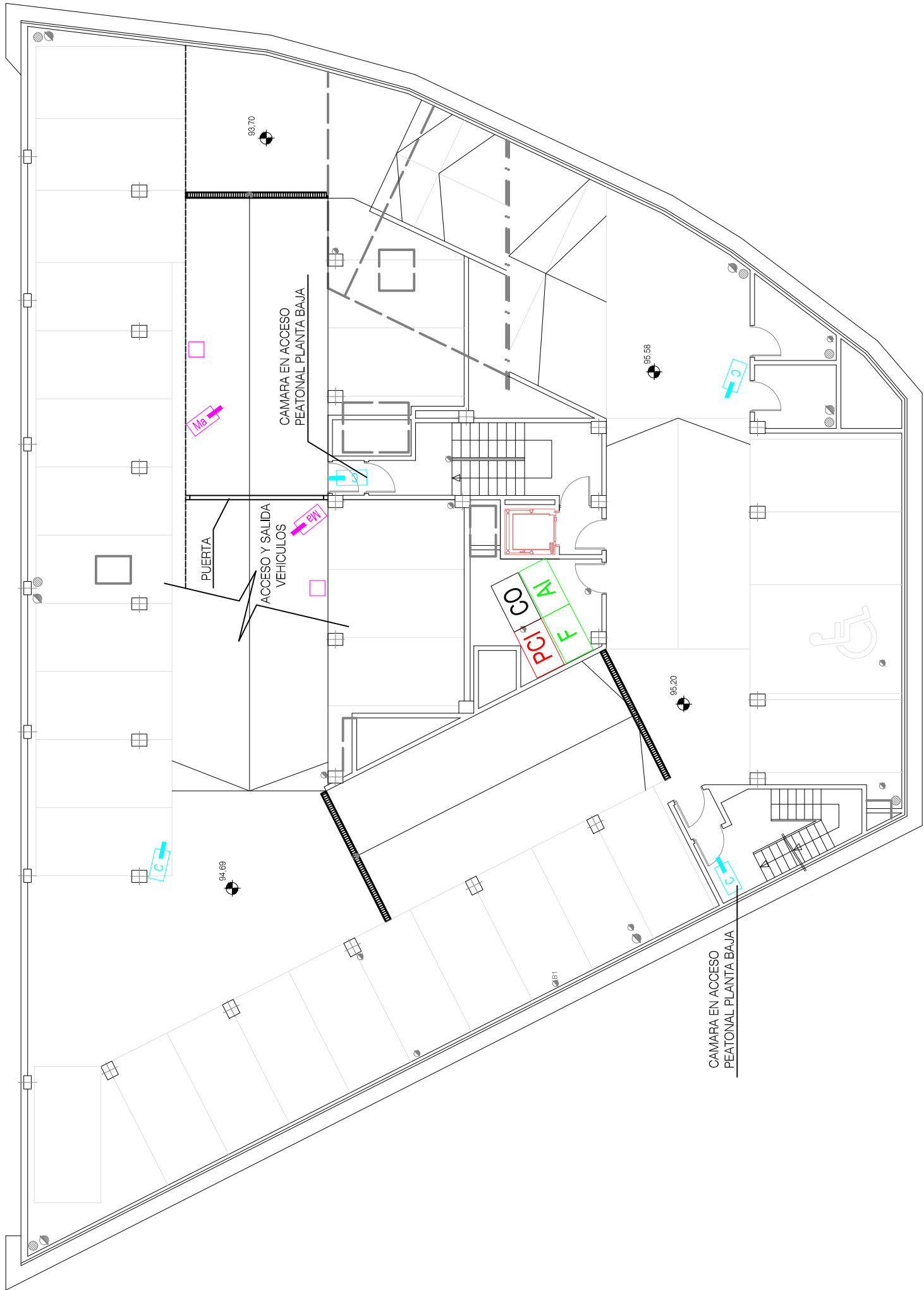
PLANTA SOTANO 1
