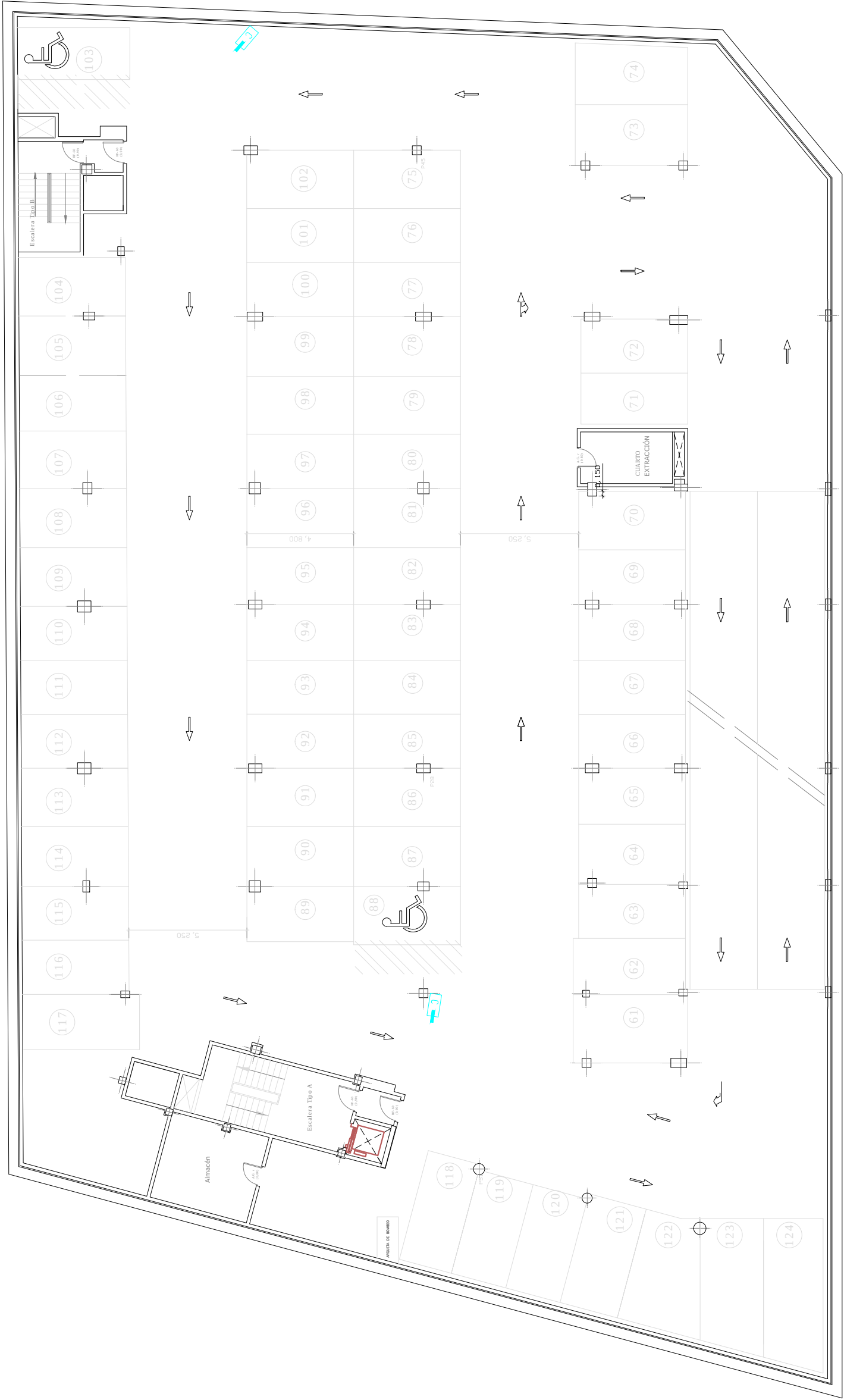
PLANTA SOTANO 3
