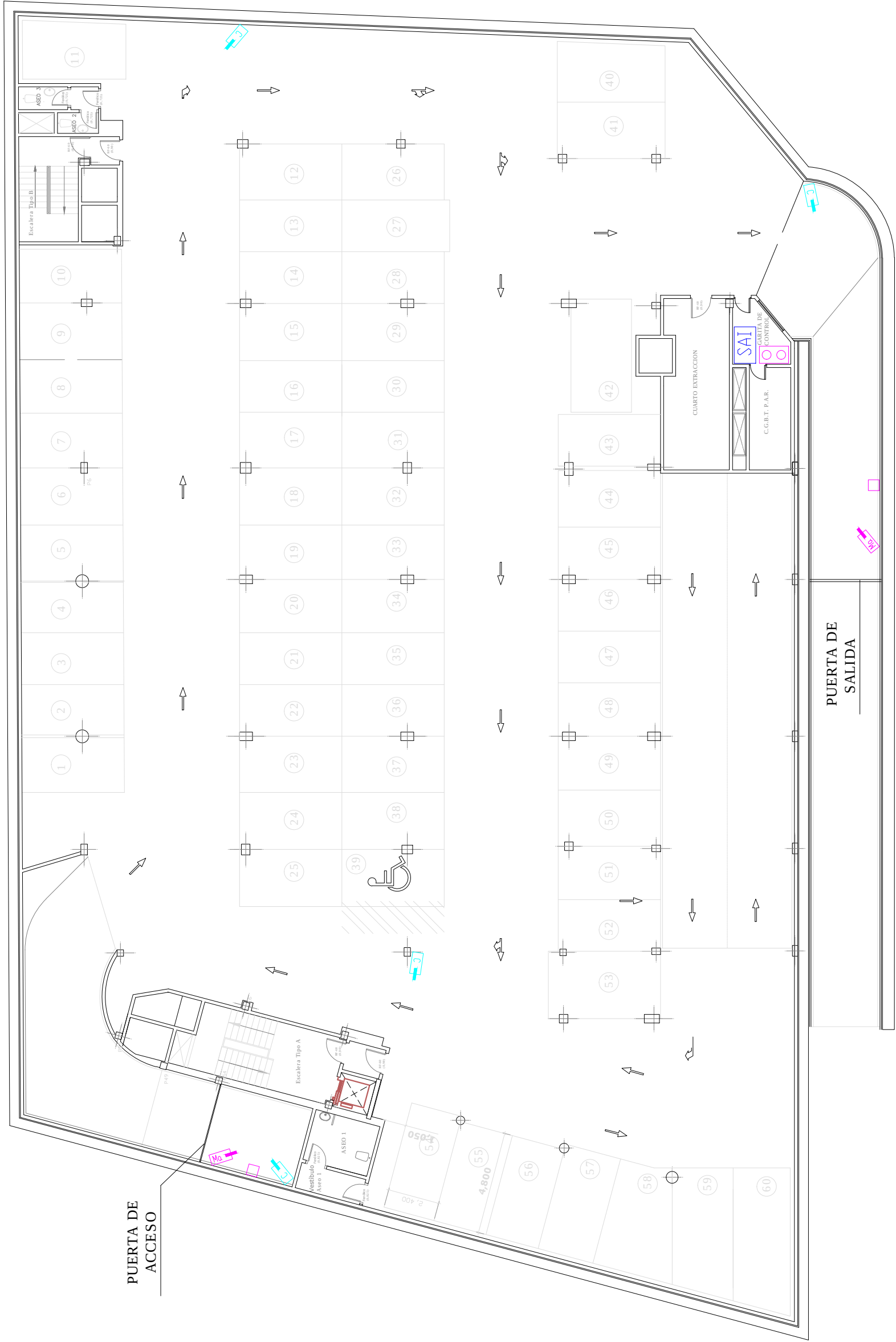
PLANTA SOTANO 2
