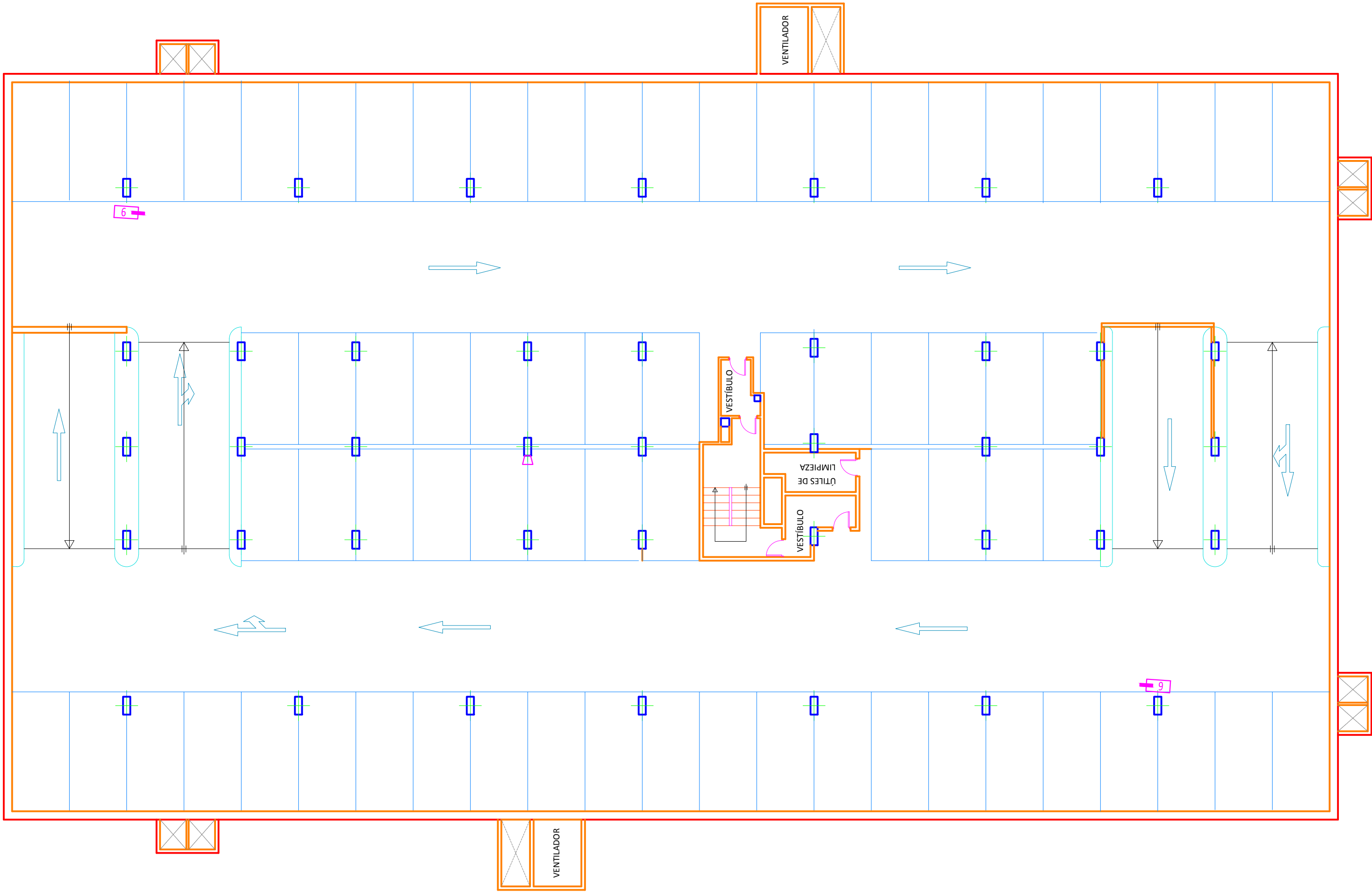
PLANTA 3 Y 4
