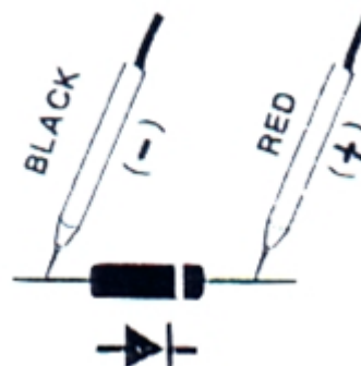
Polarización inversa.
