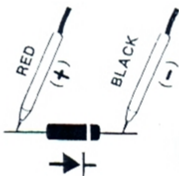
Polarización directa.
